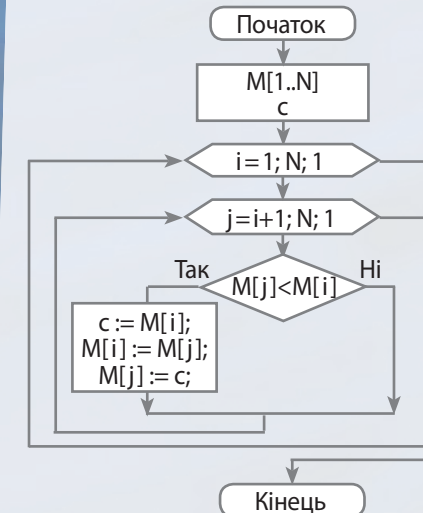
Упорядкування за зростанням (неспаданням) елементів одновимірного масиву M[1..N]
